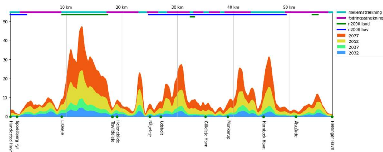
Figur 8.3: Forventet erosion i meter (y-aksen) for i forhold til vandlinjens placering år anlægsstart i referencescenariet langs strækningen (x-aksen). Erosionen er fundet som et løbende gennemsnit. Det vil sige i hvert punkt er erosionen fundet som gennemsnittet af erosionen 500 m til hver side af punktet. Øverst i figuren er projektets fodringsstrækninger (og mellemstrækninger) angivet. Lige herunder er vist hvor på kysten, der er Natura 2000-områder (grøn viser placering af Natura 2000-områder på land og blå viser marine Natura 2000-områder).
