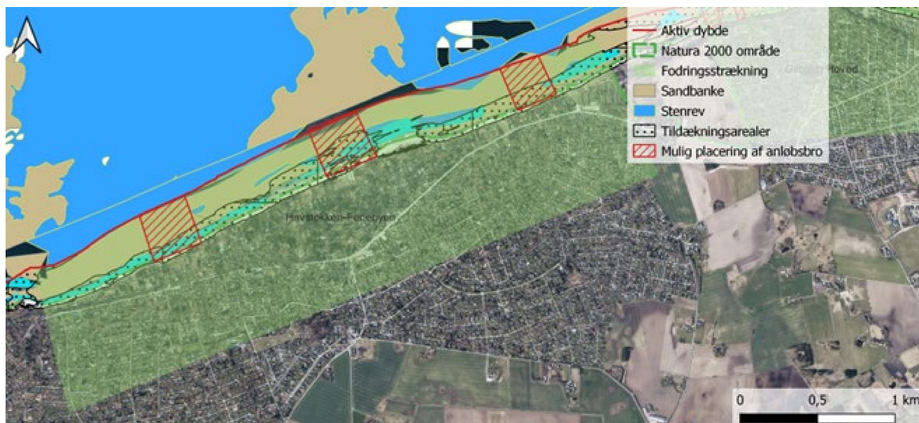
Figur 7.4: Mulig placering af anløbsbroer til indsejling af ral ved fodringsstrækningen Havstokken-Feriebyen. De mulige placeringer strækker sig fra vandlinjen og ud til den aktive dybde, ortofoto 2021.
