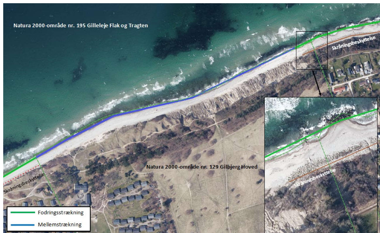
Figur 7.8: Figuren viser Natura 2000-område nr. 129 Gilbjerg Hoved med eksisterende skråningsbeskyttelse på hver side, og zoom af starten af fodringsstrækningen fra Gilbjerg Hoved til Gilleleje Havn (tyk grøn streg). Mellemstrækningen foran Natura 2000-området er vist med tyk blå streg, og fodringsstrækning Havstokken-Feriebyen med tyk grøn streg. Natura 2000-grænserne er vist med stiplet grøn streg.
